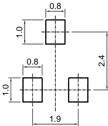
SOT-23
