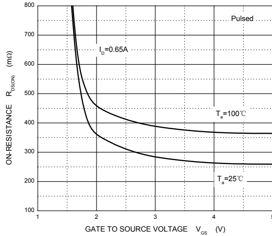
R_{DS(ON)} — V_{GS}
