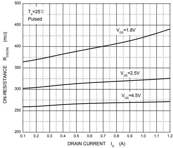
R_{DS(ON)} — I_D
