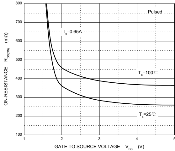
R_{DS(ON)} — V_{GS}
